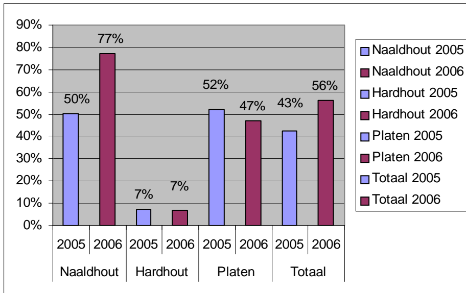
Figuur 2. Vergelijking van het aandeel afkomstig uit duurzaam beheerd gecertificeerd bos (met en zonder CoC certificaat) in 2005 en 2006 van het totale gerapporteerde volume.
